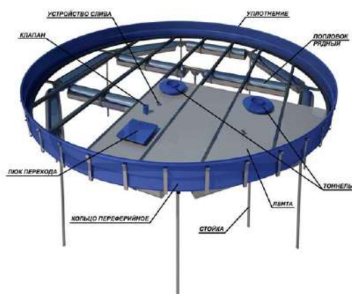
а б Рис. 1. Устройство плавающей крыши (а) и поплавков (б).
