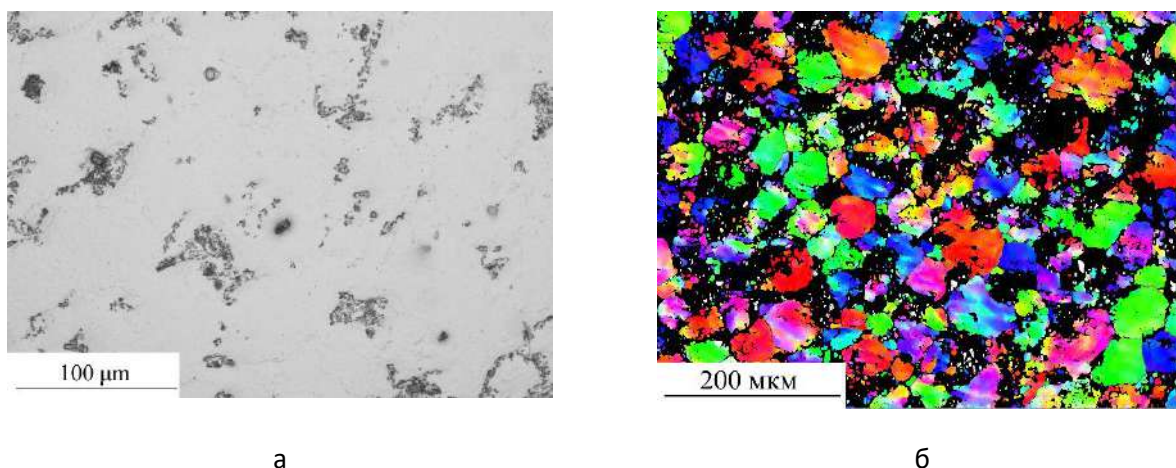
Рис. 1. Распределение частиц TiC с фракционным составом F800 (а) и зёрненная микроструктура в композите B95/2.5% TiC (б). Изображения микроструктур материалов соответствуют состоянию, полученному после гомогенизации слитка, кристаллизованного в изложнице, имеющей температуру 350 °С
